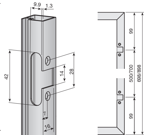
mecanizado y situación de las bisagras
