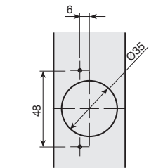
mecanizado y situación de las bisagras
