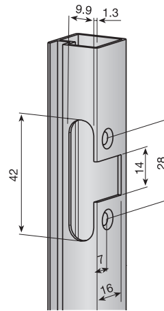
mecanizado y situación de las bisagras
