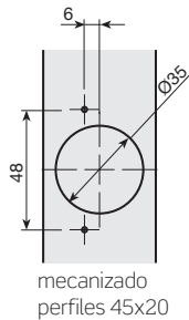
mecanizado para 2 bisagras
