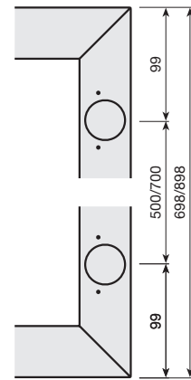
Montaje de las puertas con travesaños
