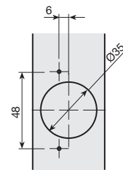
mecanizado y situación de las bisagras
